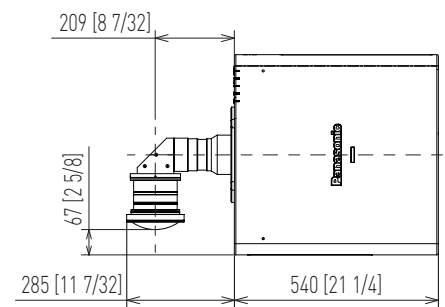
ET-D3LEU100+PT-RQ32K/PT-RZ31K/PT-RS30K
