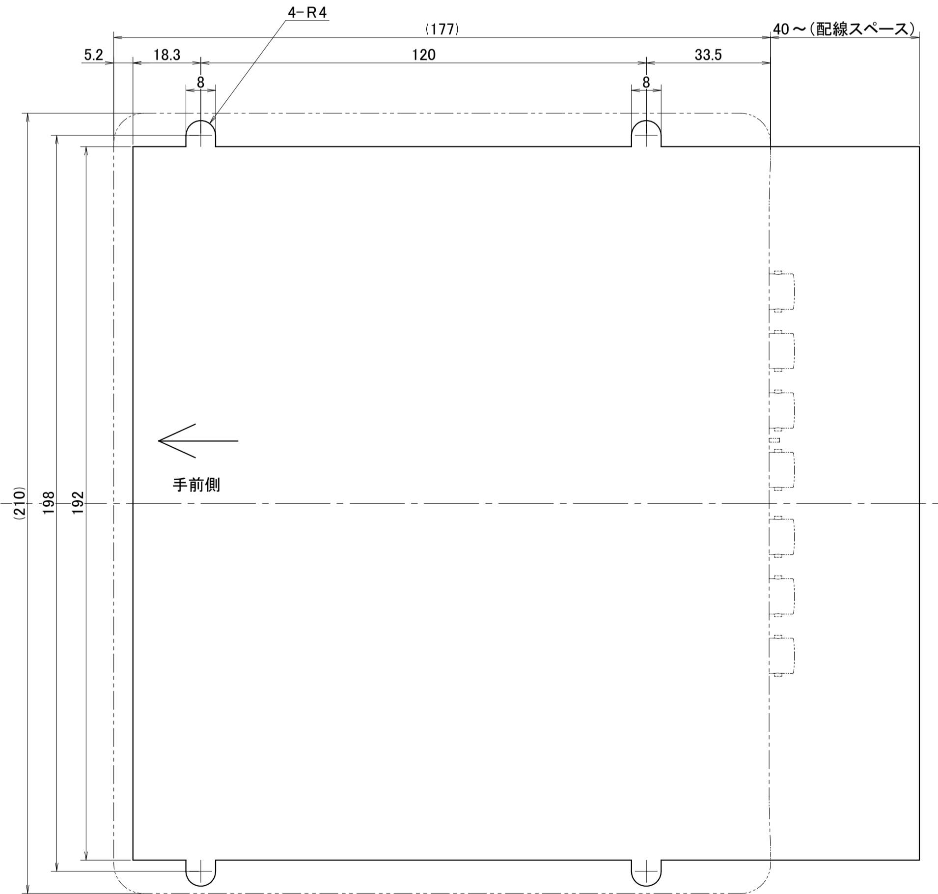
パネル埋め込み用穴あけ寸法(参考)
