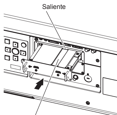
Ranura de guía Figura 2
