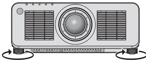
Maximal einstellbarer Bereich Einstellbare Füße: je 30 mm (1-3/16")
