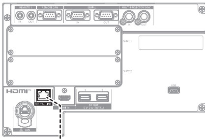
Соединительные разъемы проектора
