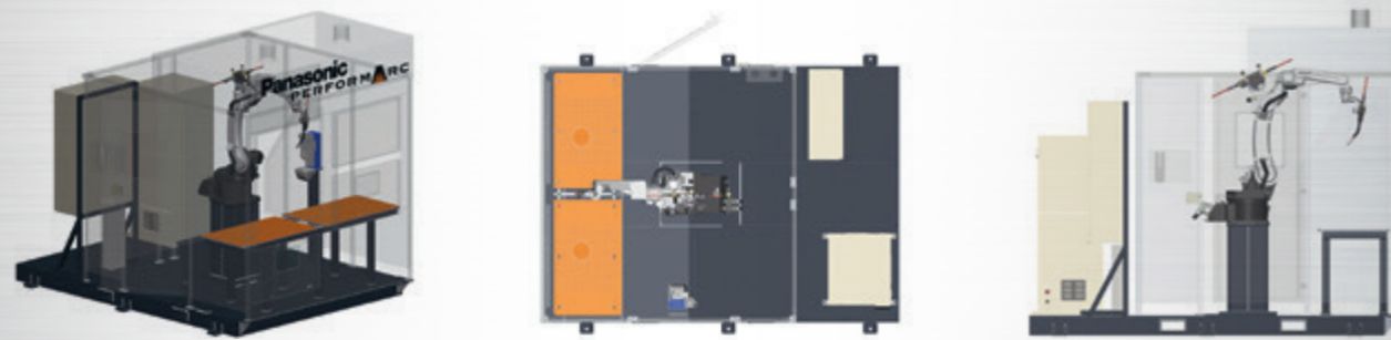
PA-TT Transparente Perspektive | PA-TT Draufsicht | PA-TT Seitenansicht
