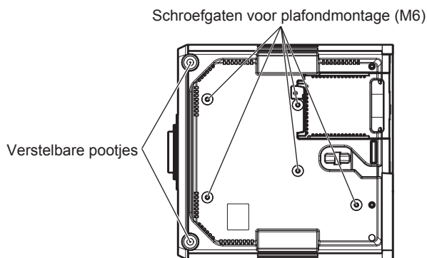
De posities van schroefgaten voor plafondmontage en verstelbare voeten
