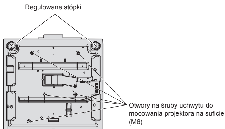
Położenie gwintowanych otworów do montażu uchwytu do mocowania na suficie oraz regulowanych stópki.
