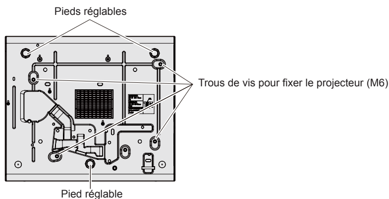
Positions des pieds réglables et des trous de vis pour fixer le projecteur
