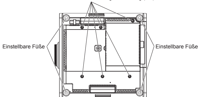
Die Positionen der Schraubenlöcher für die Aufhängevorrichtung und die einstellbaren Füße
