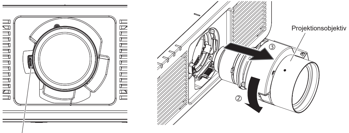
① Objektivriegelungsknopf
