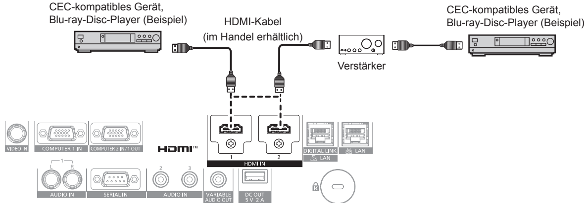
Anschlussbeispiel für ein CEC-kompatibles Gerät
