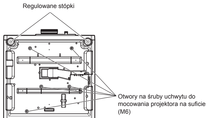
Położenie gwintowanych otworów do montażu uchwyty do mocowania na suficie oraz regulowanych stopek.
