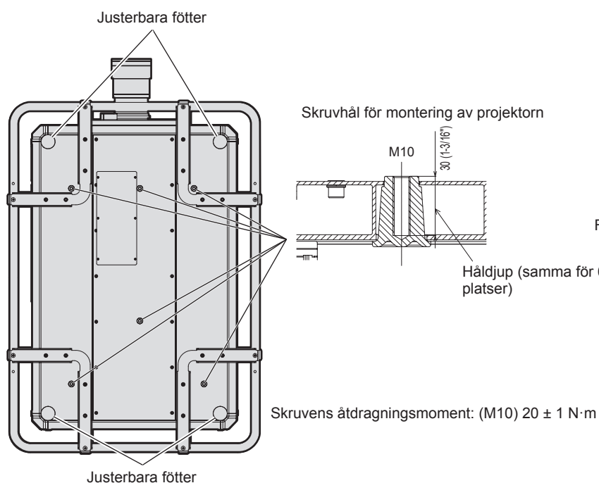
Positioner av skruvhål för montering av projektorn och justerbara fötter
