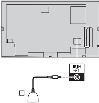
1 IR-Sensor (Standardzubehör)
