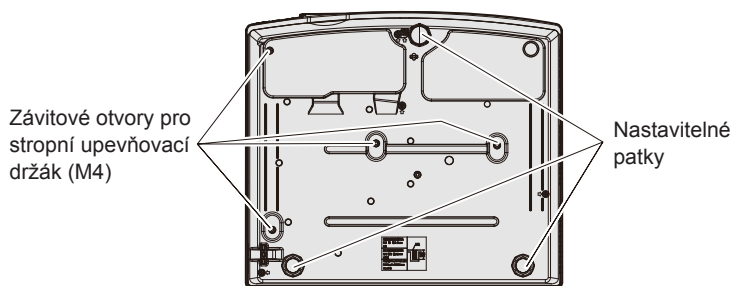
Pozice závitových otvorů pro stropní upevňovací držák a nastavitelných patek
