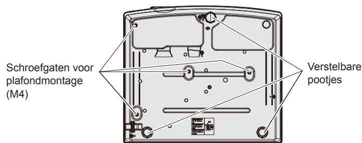
Posities van schroefgaten voor plafondmontage en verstelbare pootjes
