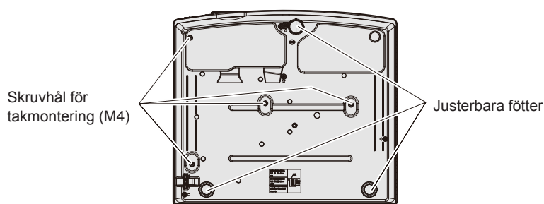
Positioner för skruvhål för takmontering och justerbara fötter
