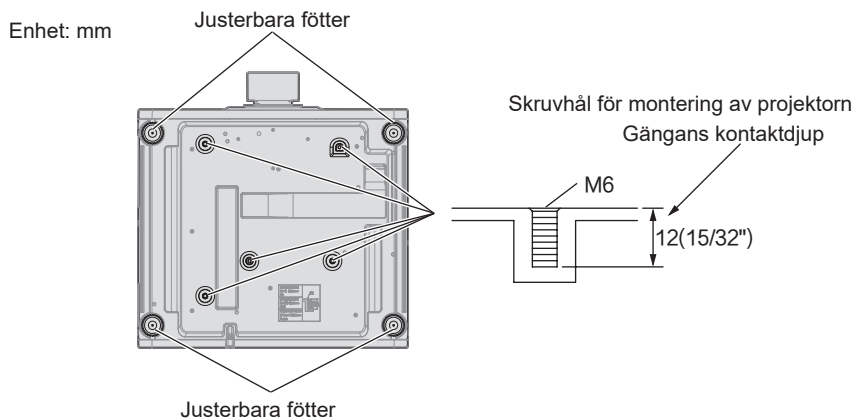
Positioner av skruvhål för montering av projektorn och justerbara fötter
