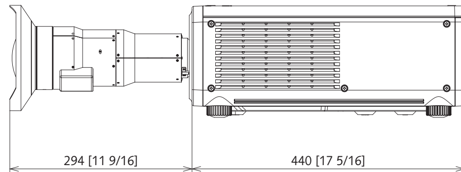
ET-DLE020+PT-RQ7/PT-RQ6/PT-RZ7/PT-RZ6
