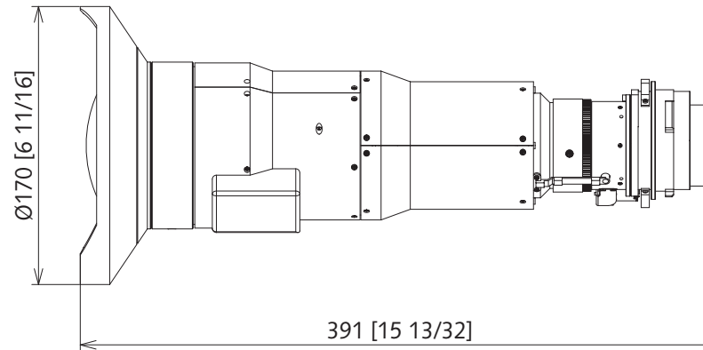
ET-DLE020
