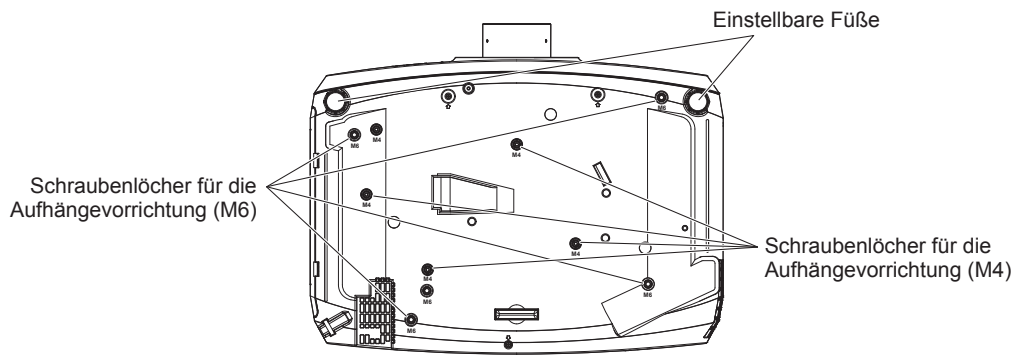
Die Positionen der Schraubenlöcher für die Aufhängevorrichtung und die einstellbaren Füße
