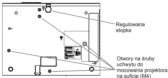
Położenie gwintowanych otworów do montażu uchwytu do mocowania na suficie oraz regulowanych stopek
