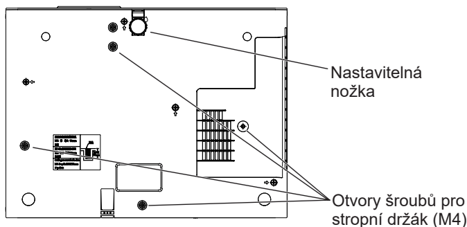
Polohy otvorů se závitem pro stropní upevňovací držák a poloha nastavitelná nožka
