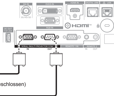
Anschlüsse des dritten Projektors
