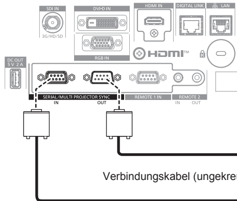
Anschlüsse des vierten Projektors
