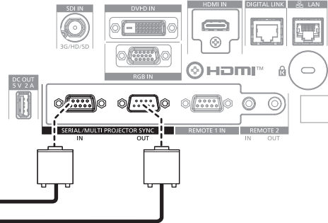
Anschlüsse des dritten Projektors
