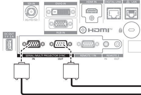
Anschlüsse des vierten Projektors
