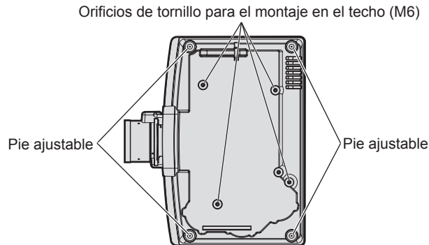
Posiciones de los orificios de tornillo para el montaje en el techo y los pies ajustables
