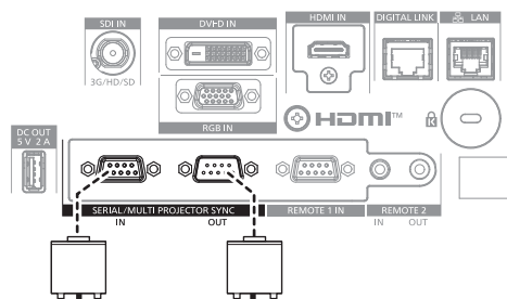
Terminali di collegamento del primo proiettore
