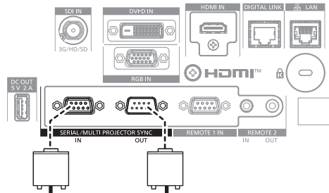
Terminali di collegamento del quarto proiettore
