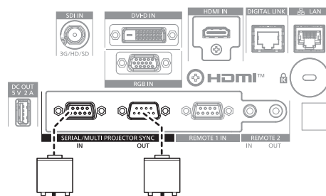
Terminali di collegamento del secondo proiettore
