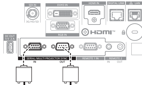
Terminali di collegamento del terzo proiettore
