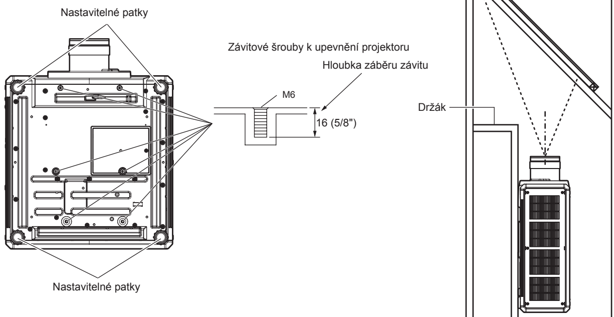
Pozice závitových otvorů pro upevnění projektoru a nastavitelných patek
