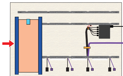
Vista trasera del cabinet
