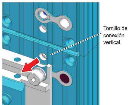
Vista ampliada de las piezas de conexión
